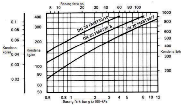
DN15 FMBT30
