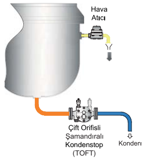
Ceketli kazan
