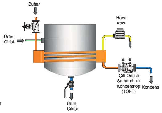
Evaporatör
